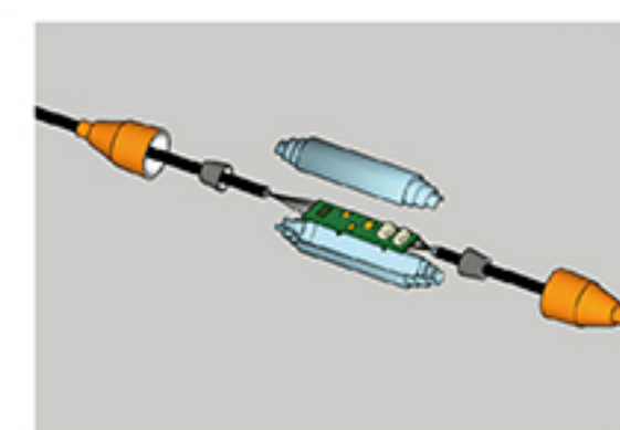
电缆剖析图
